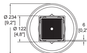
Dimensiones: vista cenital
