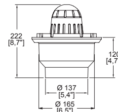
Dimensiones: vista lateral
